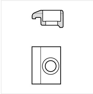
Spannstück CKX 20-145
